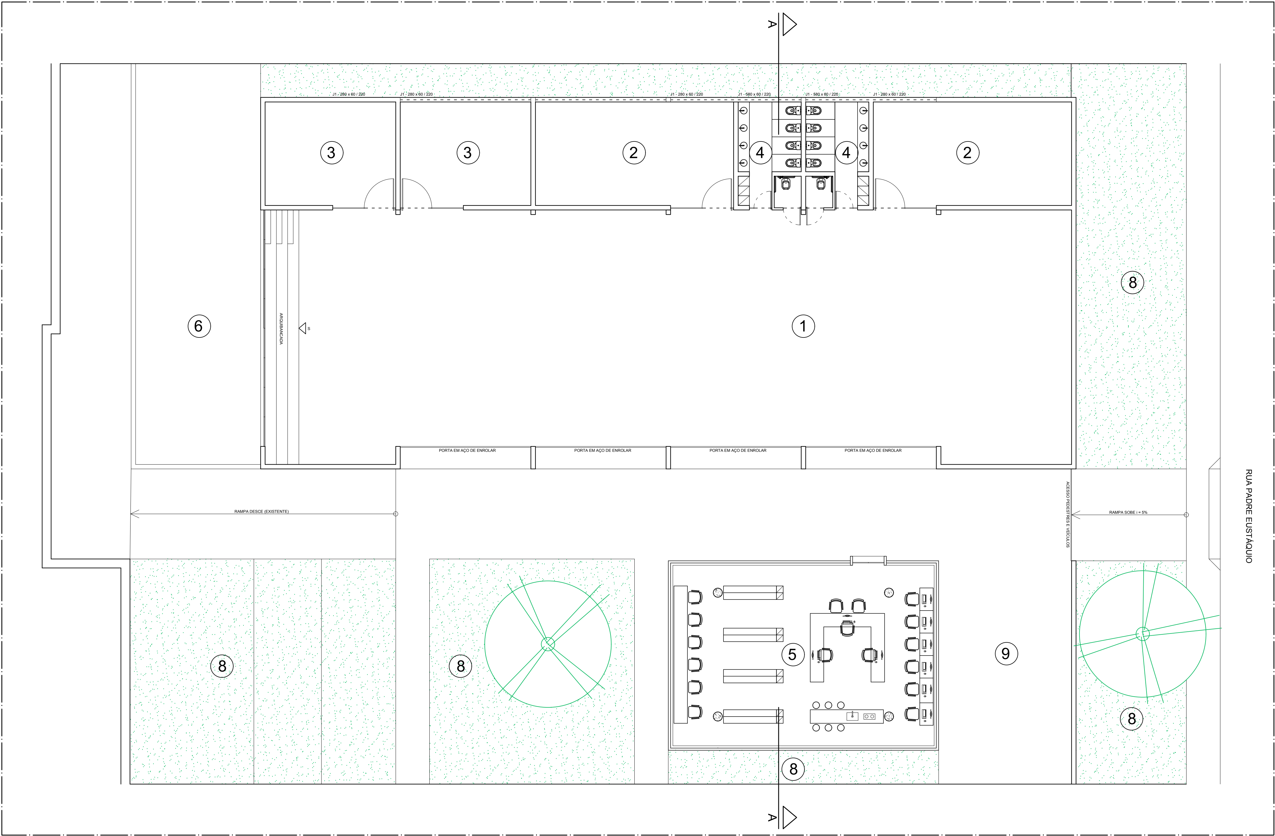
PLANTA 1º PAVIMENTO ESCALA 1:100
